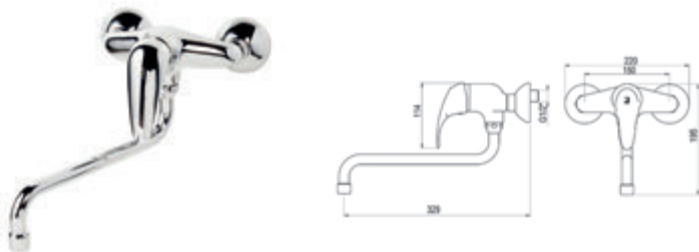
ALFA / Grifo de cocina mural / Wall kitchen tap
